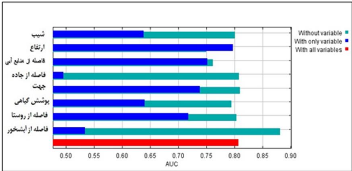
شکل ۲- نتایج روش جک نایف برای پیش‌بینی مهمترین متغیرهای مؤثر بر پراکنش آهو در منطقه مورد مطالعه
