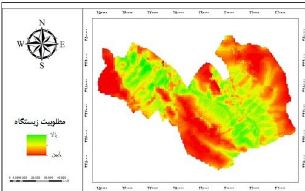
شکل ۳- مدل توزیع پیوسته کنونی آهو در منطقه حفاظت شده کالمند-بهداران
